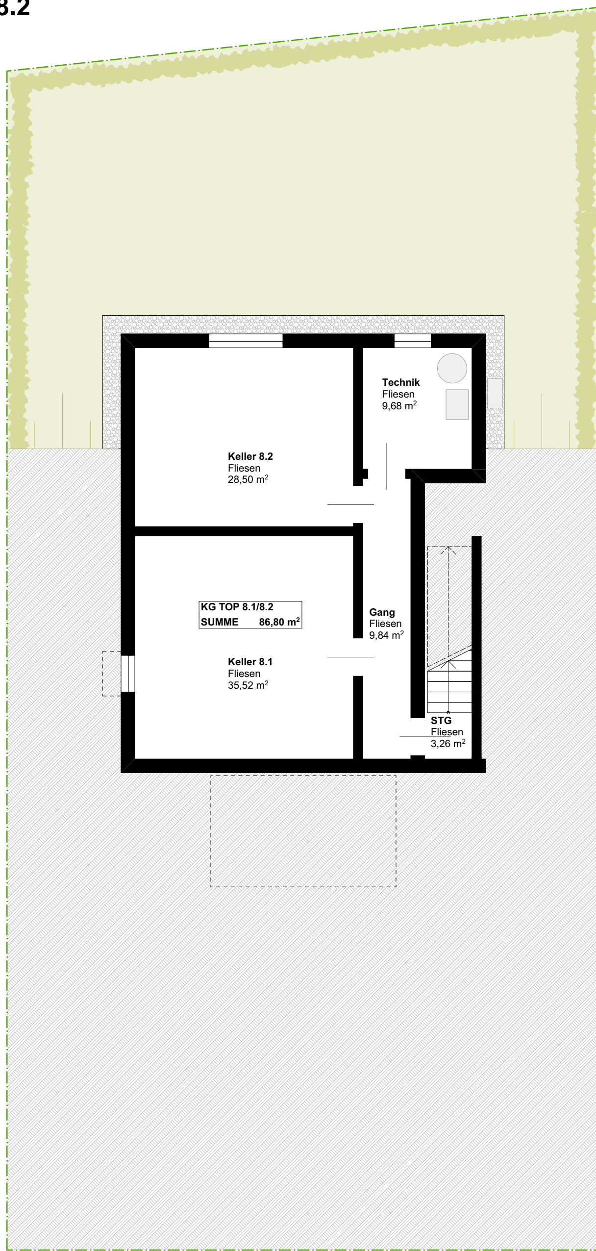
Kellergeschoss M1:100
