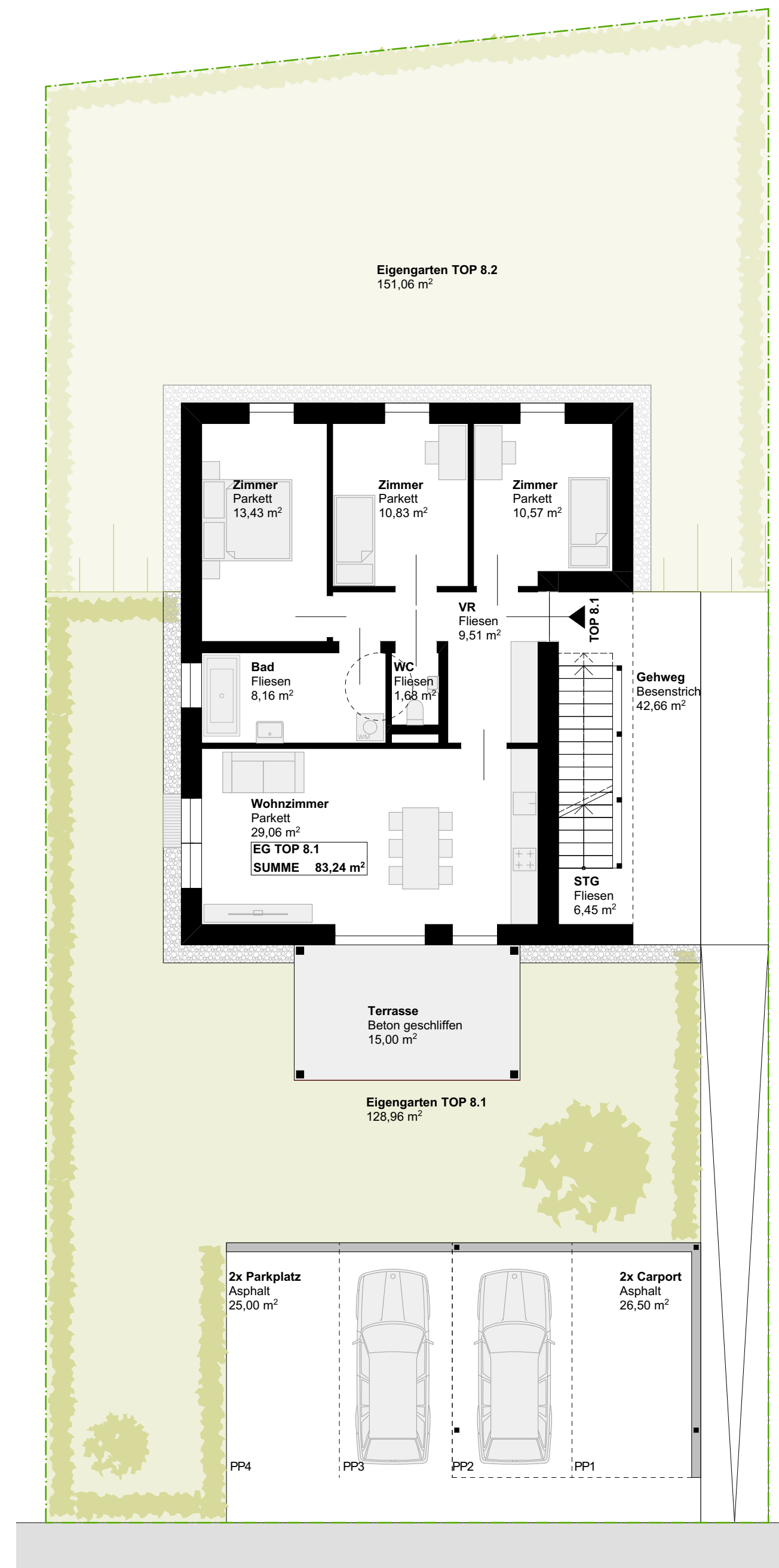
Erdgeschoss M1:100
