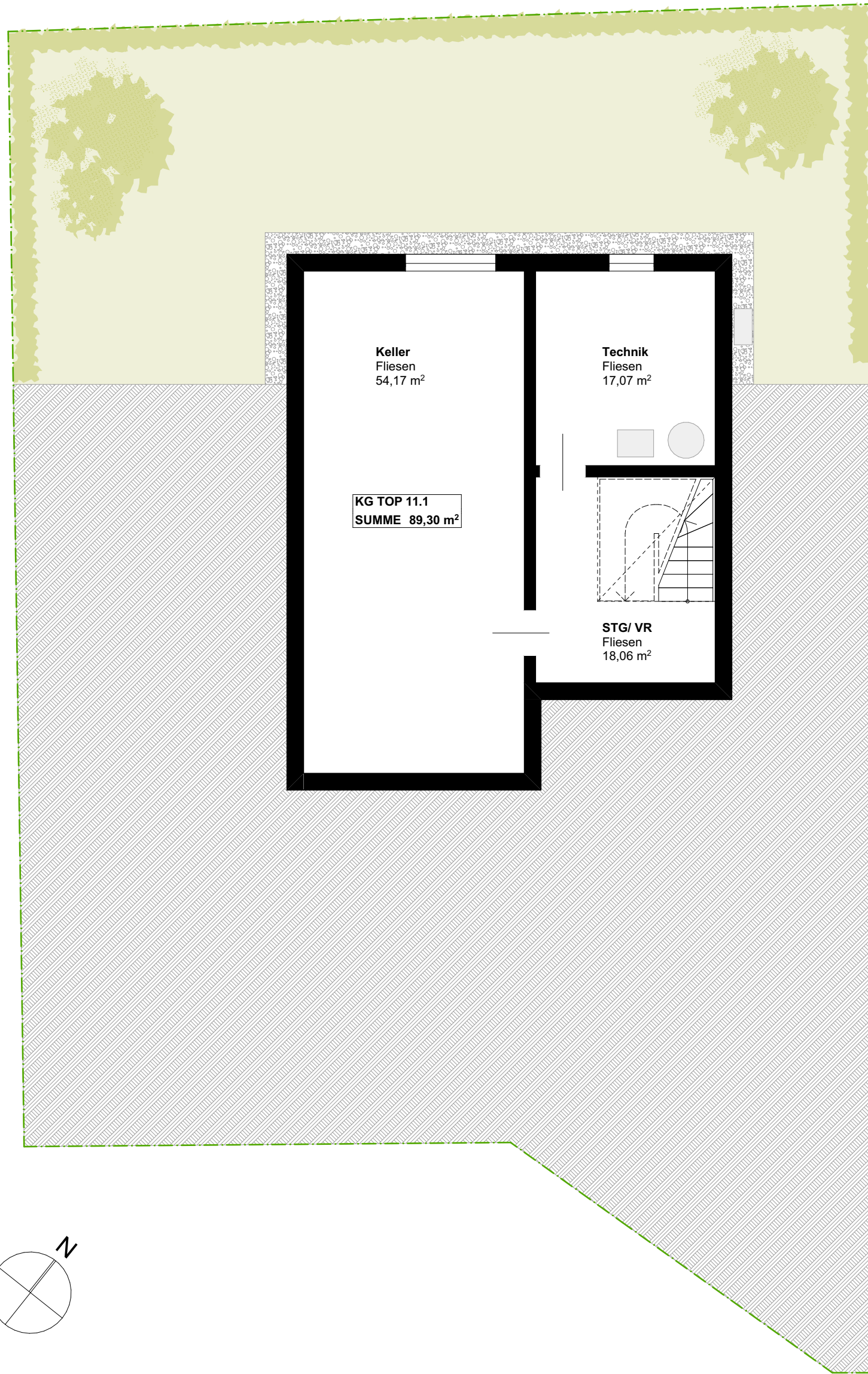
Kellergeschoss M1:100
