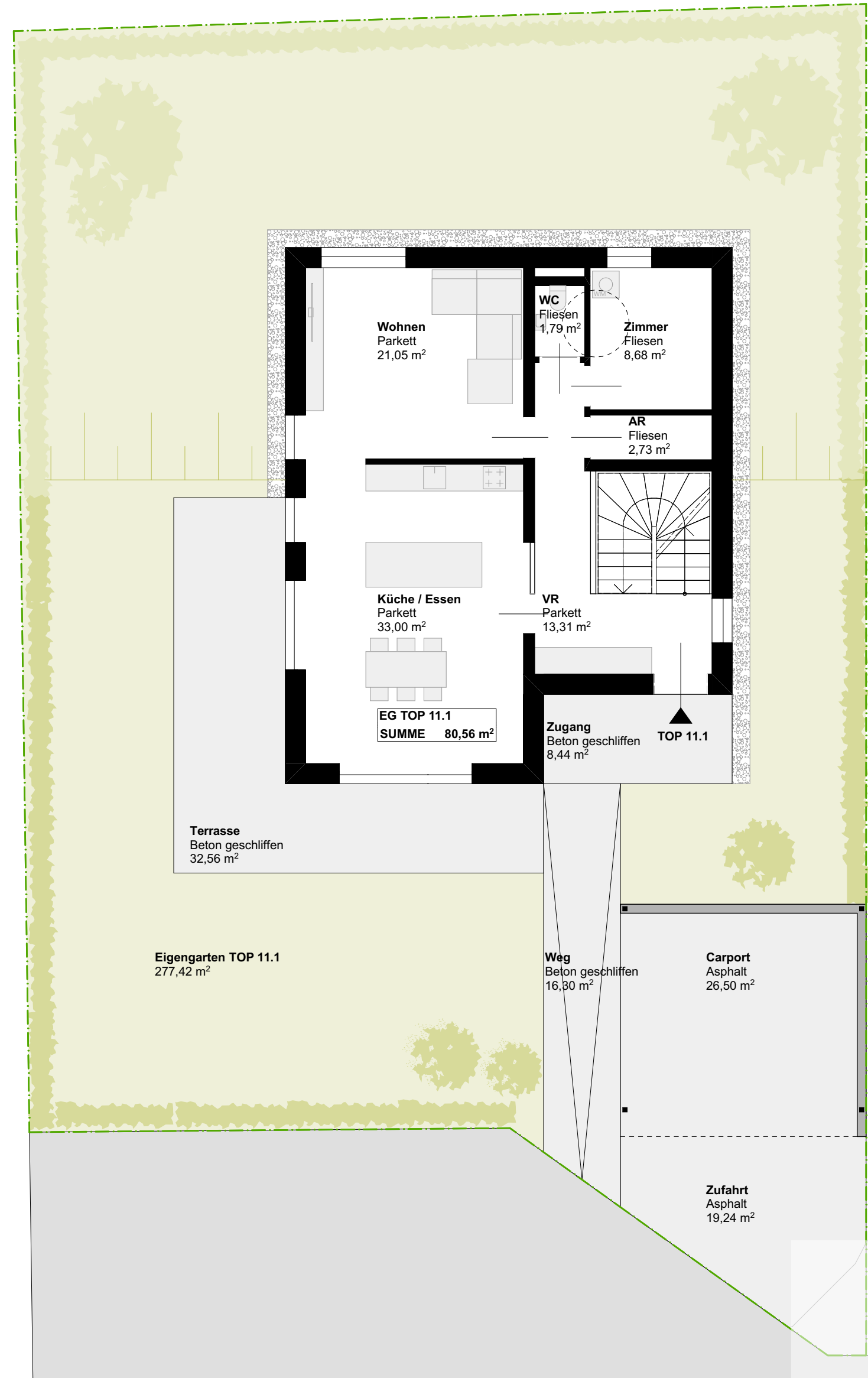
Erdgeschoss M1:100
