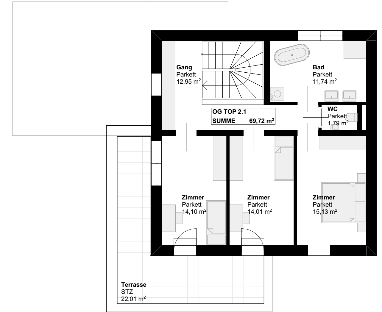
1. Obergeschoss M1:100
