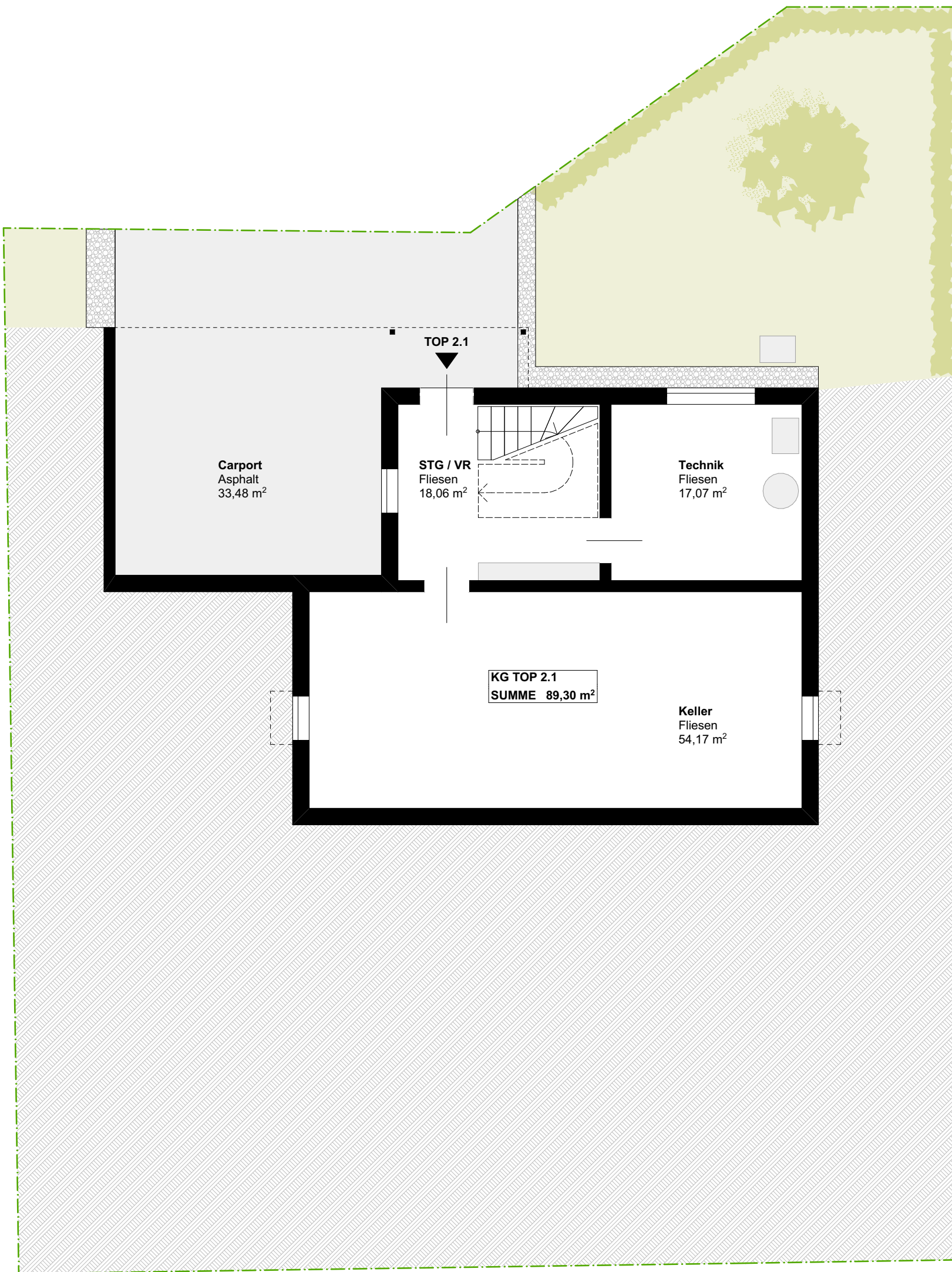
Kellergeschoss M1:100
