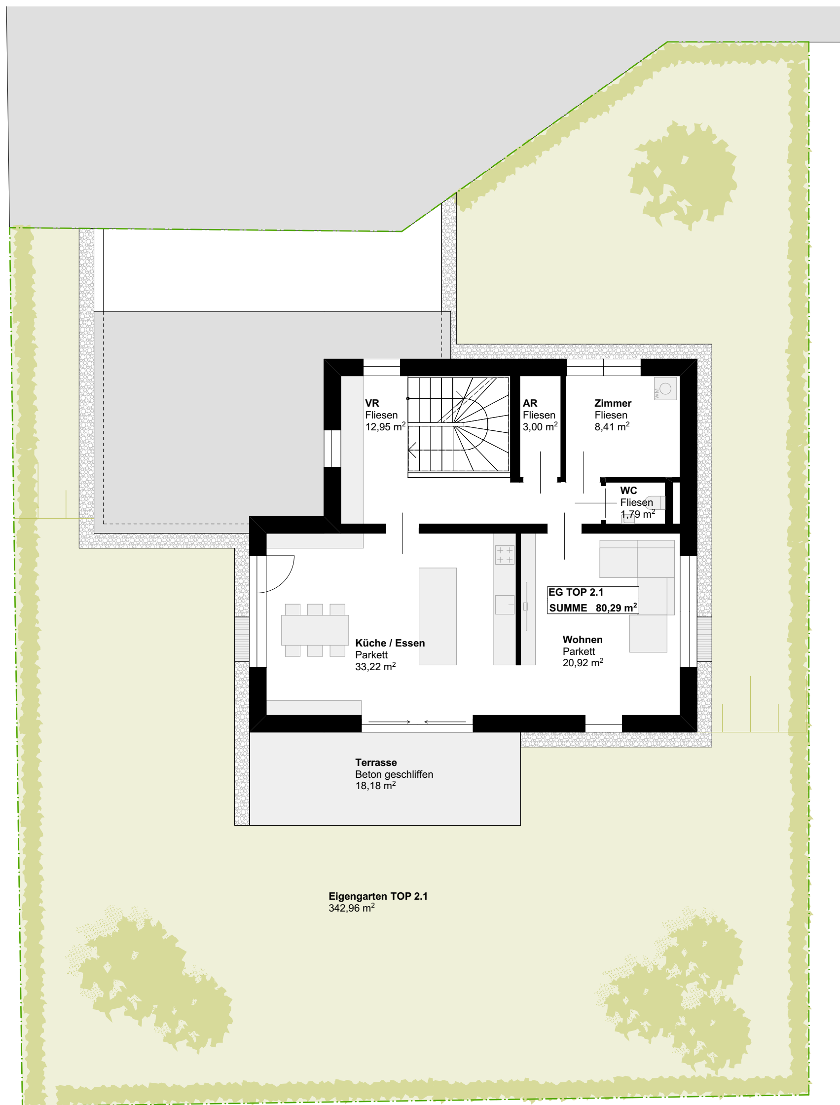
Erdgeschoss M1:100
