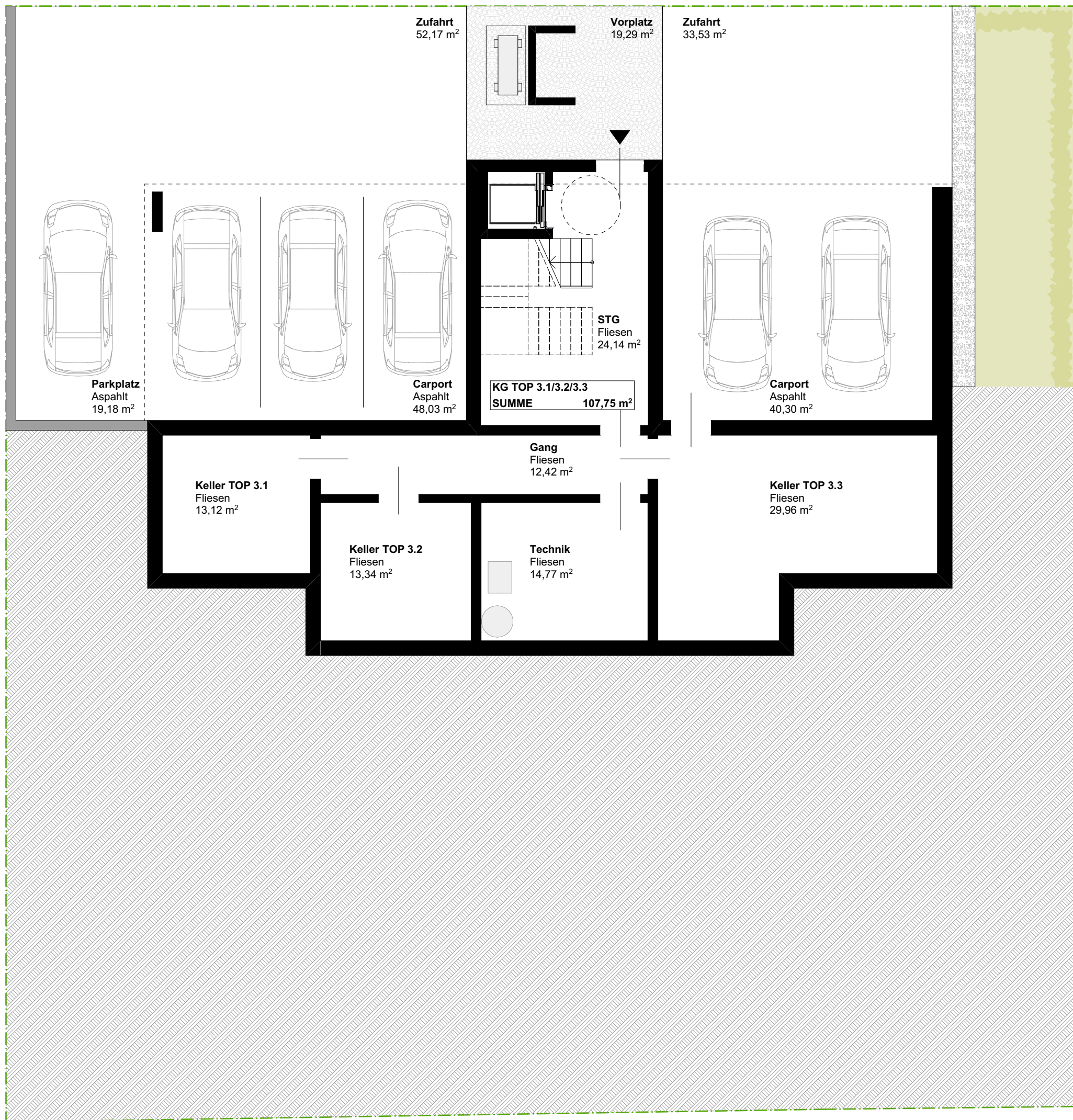
Kellergeschoss M1:100
