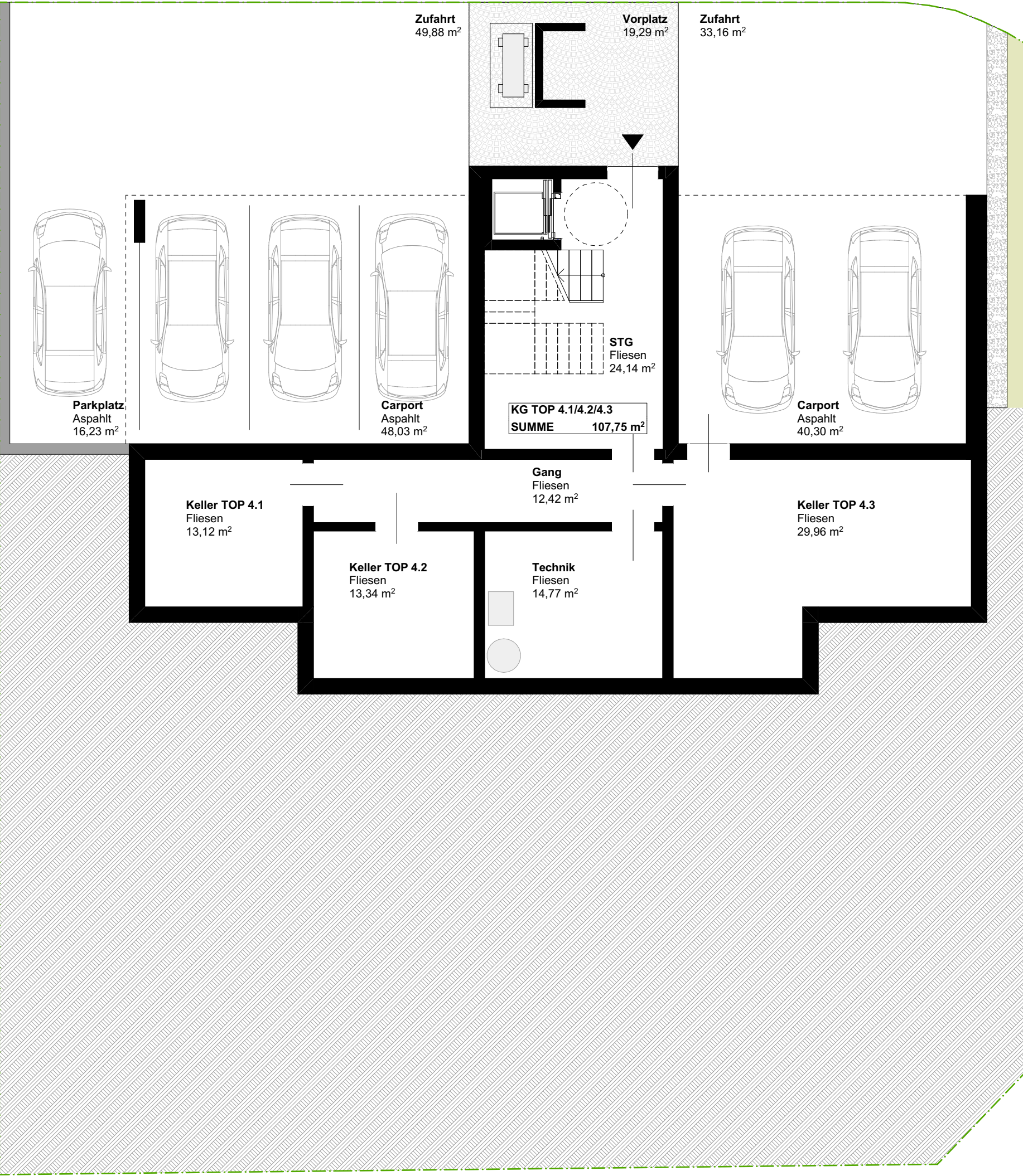
Kellergeschoss M1:100
