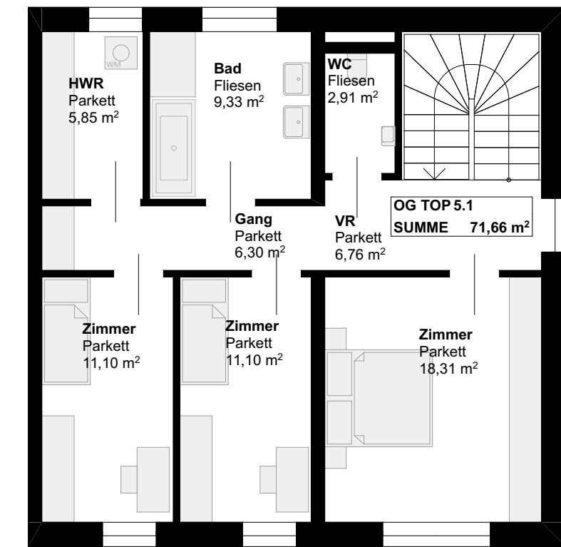
1. Obergeschoss M1:100
