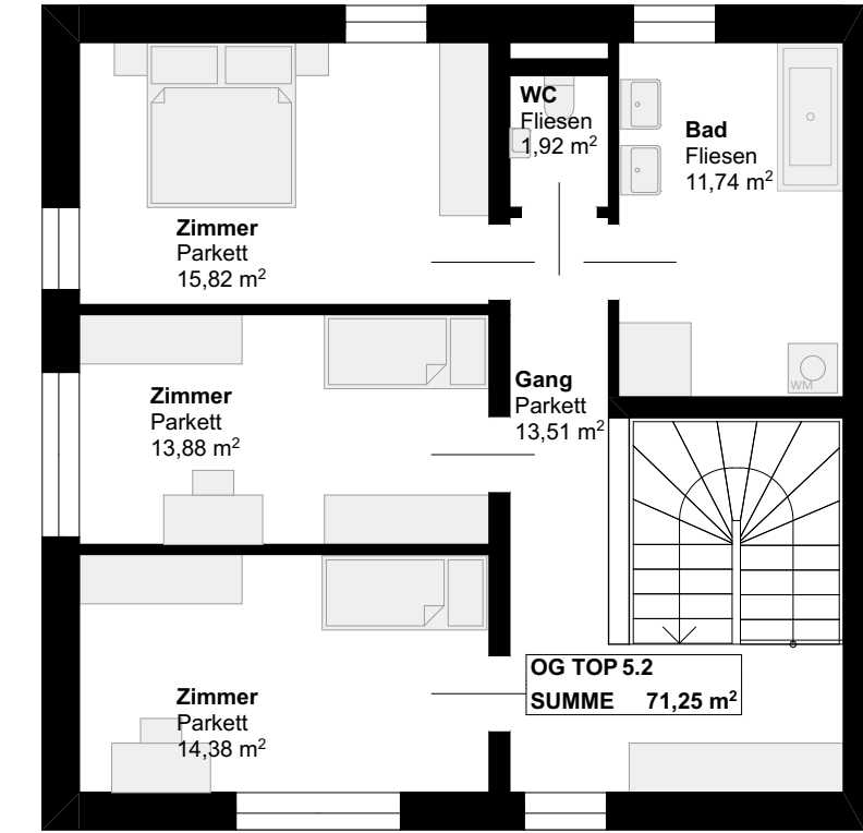
1. Obergeschoss M1:100
