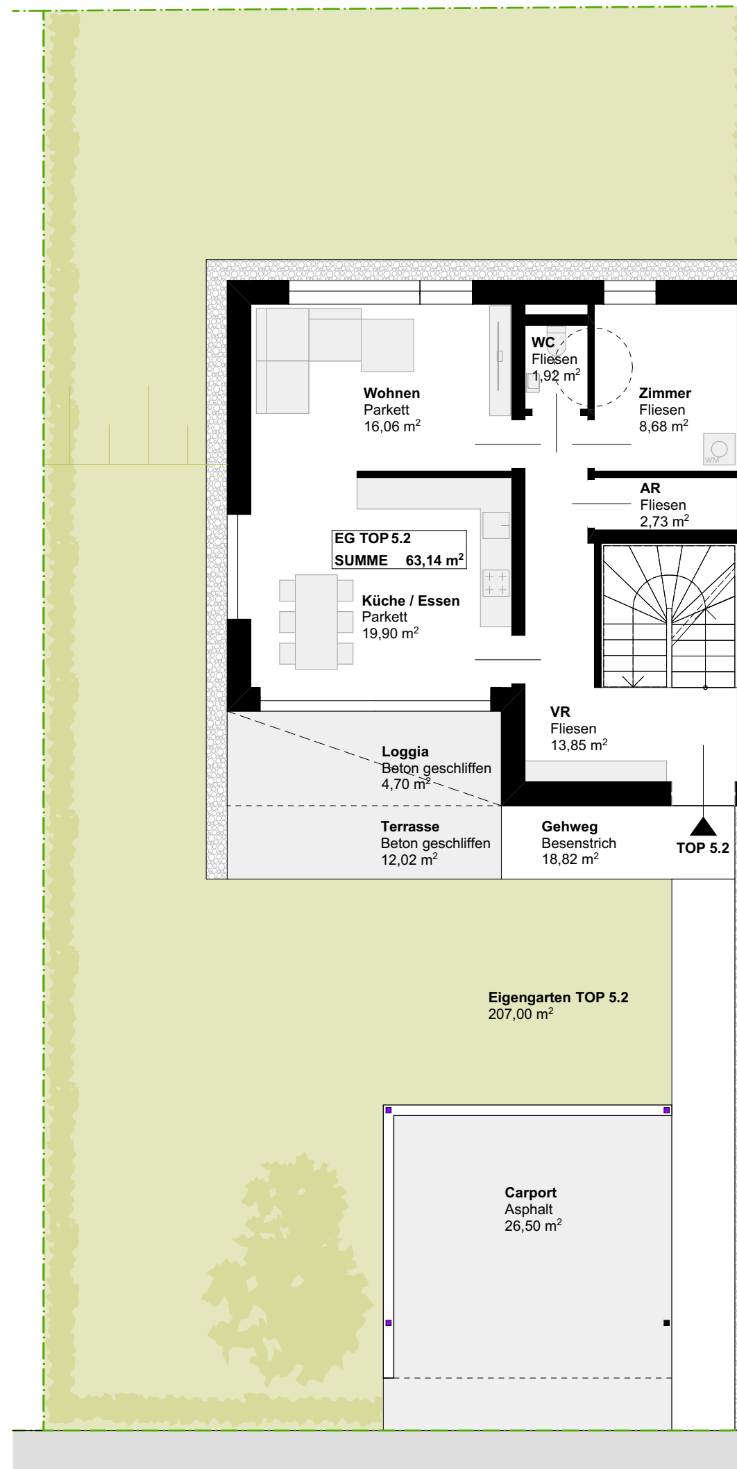
Erdgeschoss M1:100
