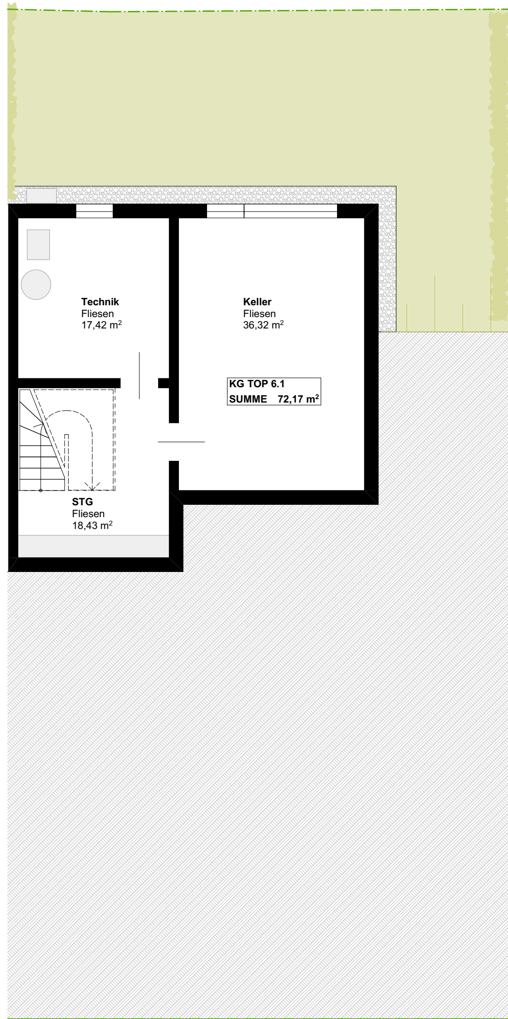
Kellergeschoss M1:100
