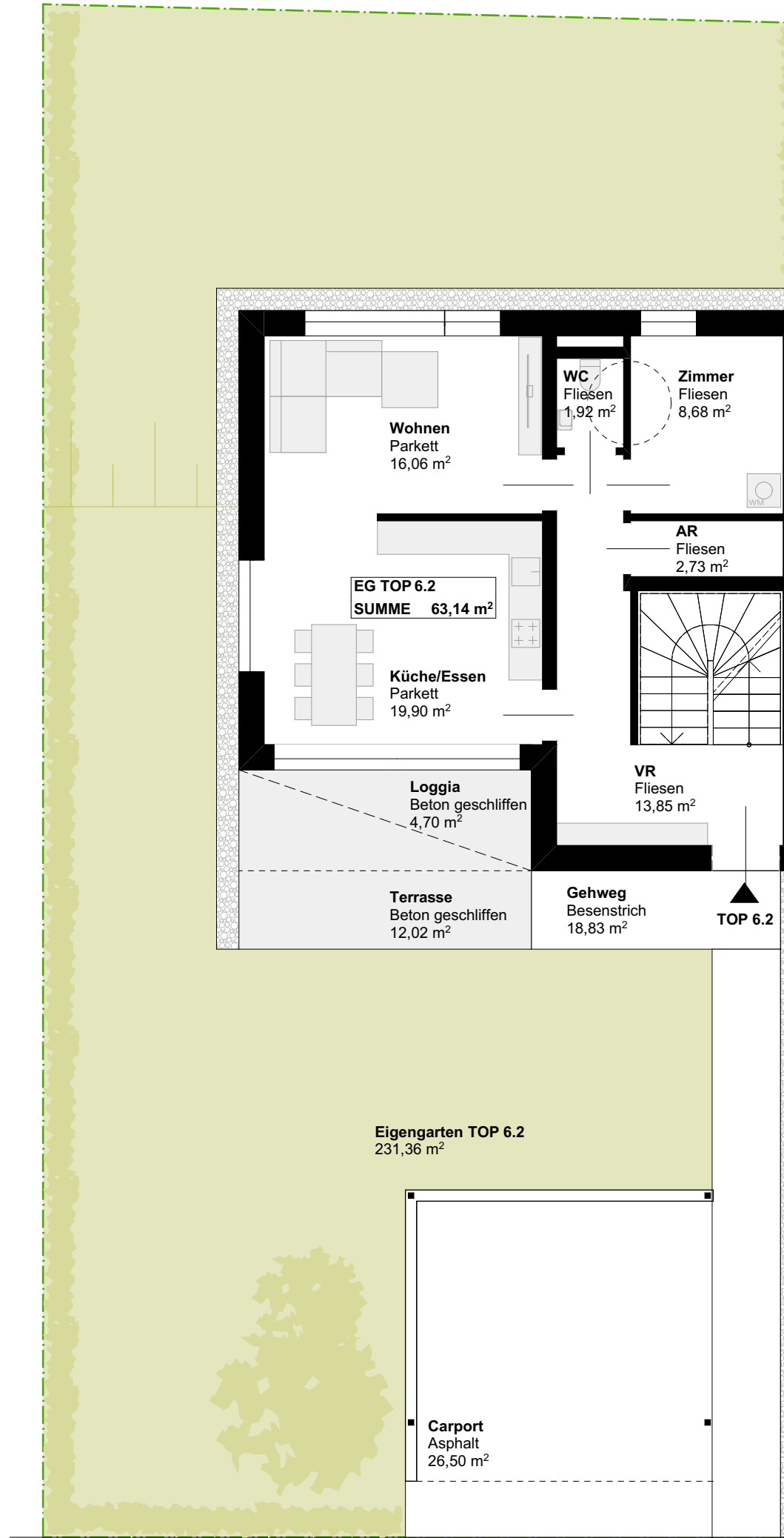
Erdgeschoss M1:100
