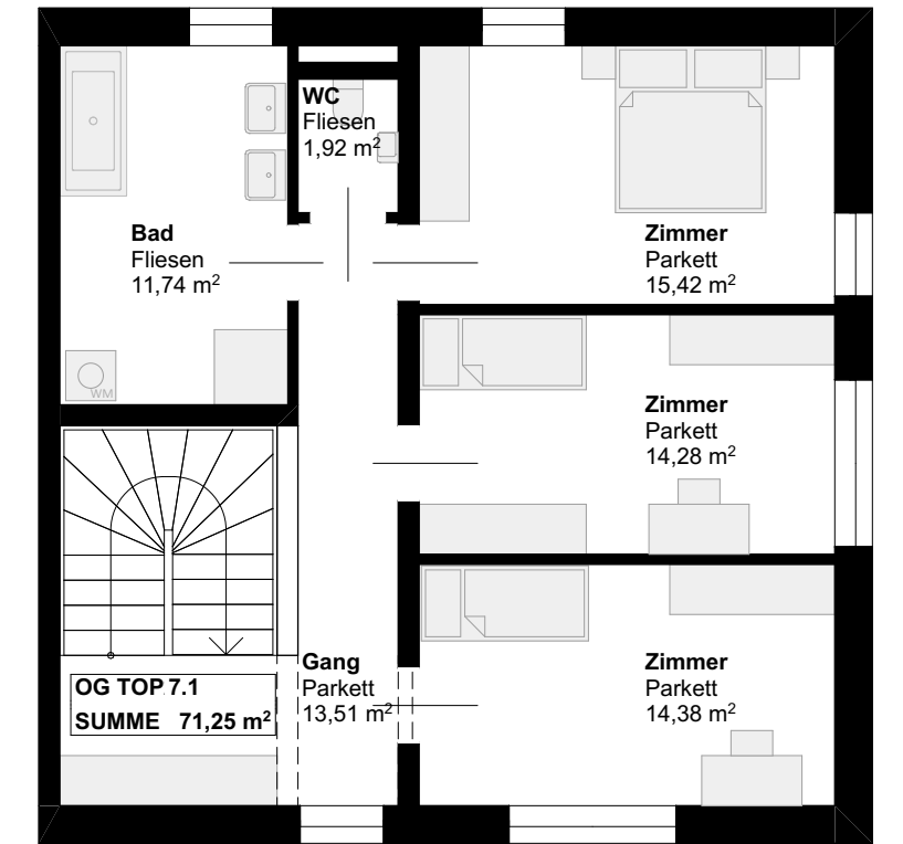
1. Obergeschoss M1:100
