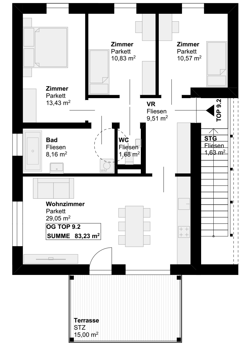
1. Obergeschoss M1:100
