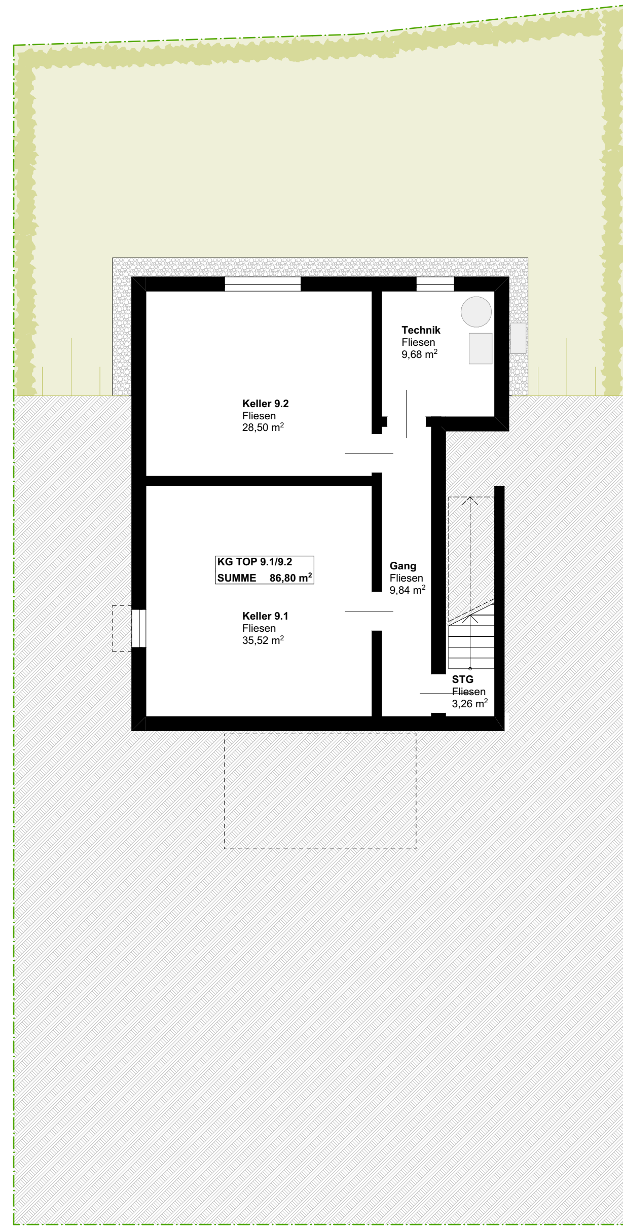
Kellergeschoss M1:100
